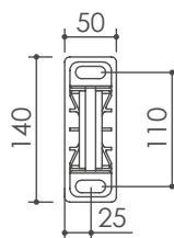
Staffa attacco a parete/soffitto
