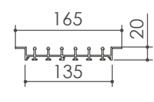
Profilo inferiore incassato 6 vie
