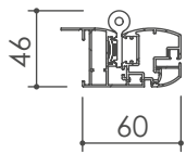
Cerniera con molla classica
