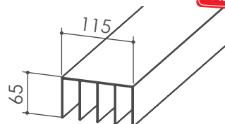
Profilo compensatore 5 vie
