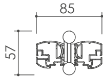
Cerniera con molla saloon
