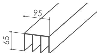
Profilo compensatore 4 vie
