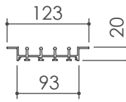
Profilo inferiore incassato 4 vie
