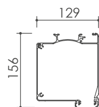
Cassonetto Square
