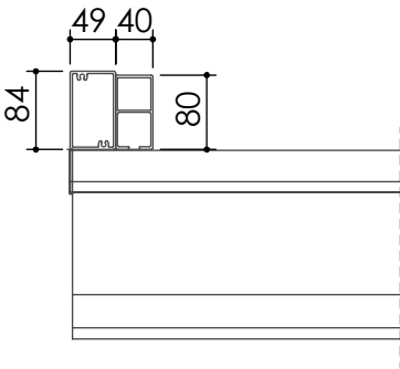
SEZIONE FRONTALE
