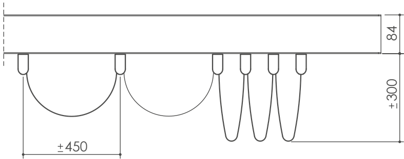
SEZIONE LATERALE CON PROFILO 80/40
