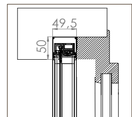
BORA TOP INCAS DOPPIA MIDI 50/50
