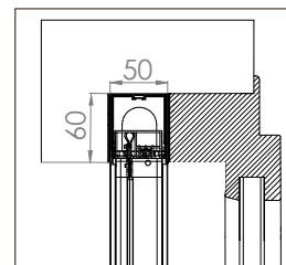
BORA TOP INCAS DOPPIA STANDARD 20/20
