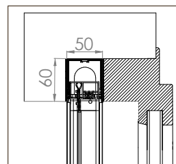
BORA TOP INCAS DOPPIA STANDARD 50/50
