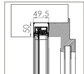
BORA TOP INCAS DOPPIA MIDI 35/35
