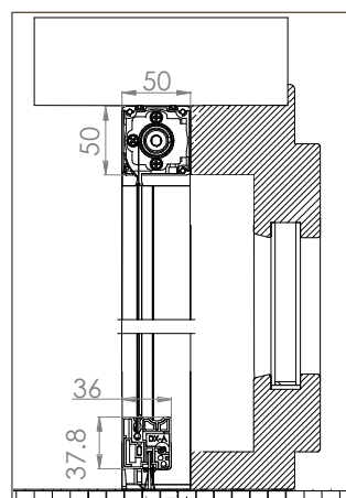
IRINA INSTALLAZIONE IN LUCE
