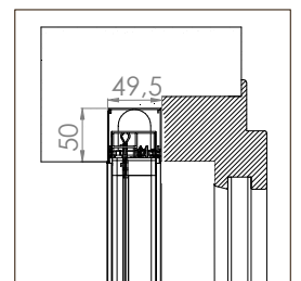
BORA INCAS DOPPIA MIDI 20/20
