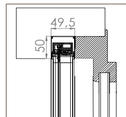
BORA TOP INCAS MIDI 50/35
