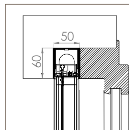
BORA INCAS DOPPIA STANDARD 20/20
