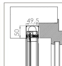
BORA INCAS DOPPIA MIDI 35/35
