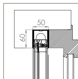
BORA INCAS DOPPIA STANDARD 35/35
