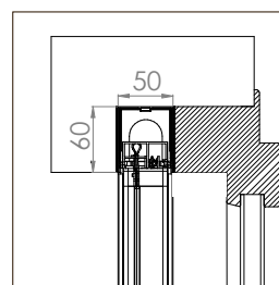
BORA INCAS DOPPIA STANDARD 50/50
