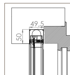
BORA INCAS DOPPIA MIDI 50/50
