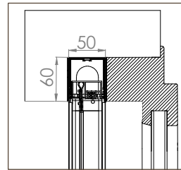
BORA TOP INCAS DOPPIA STANDARD 35/35
