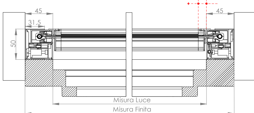
Compensazione fino a 6 mm
