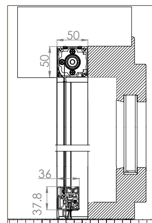
IRINA INSTALLAZIONE A INCASSO
