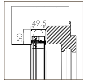
BORA INCAS MIDI 50/35
