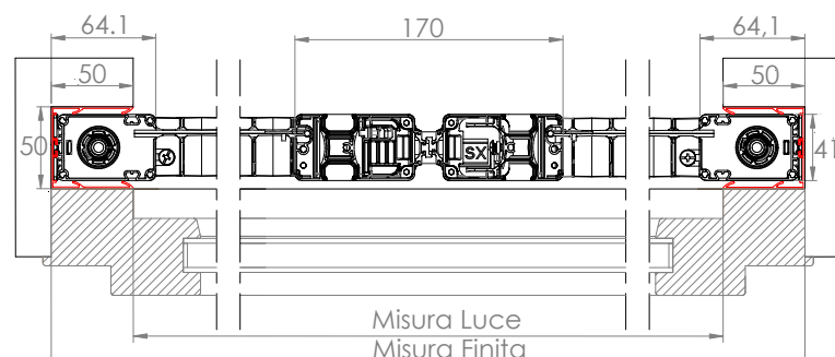
BORA INCAS DOPPIA STANDARD 50/50
