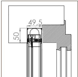
BORA INCAS SR MIDI 35
