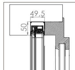
BORA TOP INCAS DOPPIA MIDI 20/20
