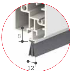
Barra maniglia con profilo portaspazzolino telescopico (fino a 8 mm)
