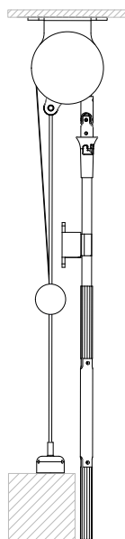
Tendicavo basso per fissaggio a pavimento.
