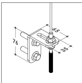
Staffe in acciaio AISI 304 76x65x35 mm
