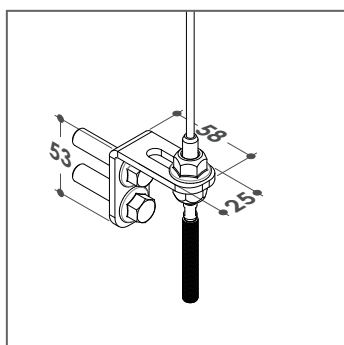
Staffe in acciaio AISI 304 53x58x25 mm
