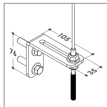
Staffe in acciaio AISI 304 76x105x35 mm
