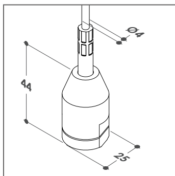
Cilindro tendicavo in acciaio inox AISI 316.
