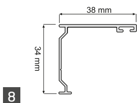
8 Profilo laterale prima anta
