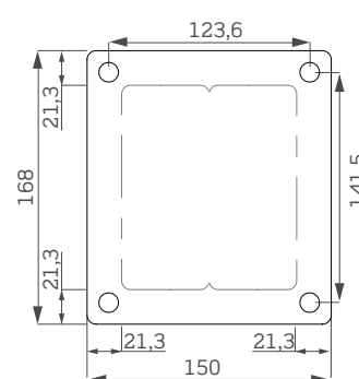
Piastra Mope di ancoraggio a terra
